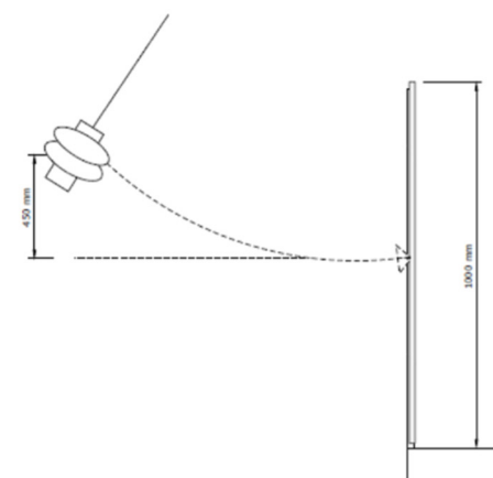
Fig. 6. Pendelprøving av Metode C.
