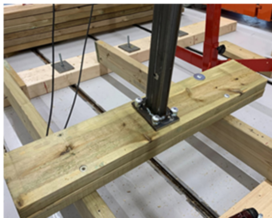
Figur 18 Alternativ løsning for toppmontert stolpe, trukket inn på trebjelkelag, for eksempel takterrasse med tilfarergulv. Plankene kan felles ned i bjelkene. Se vedlegg C, prøveoppstilling G for detaljer
