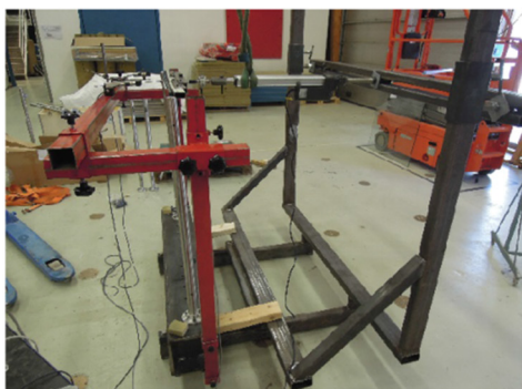
Fig. 2. Rekkverksprøverigg med aktuator og lastpåføringsbjelke ved prøving av Metode B.
